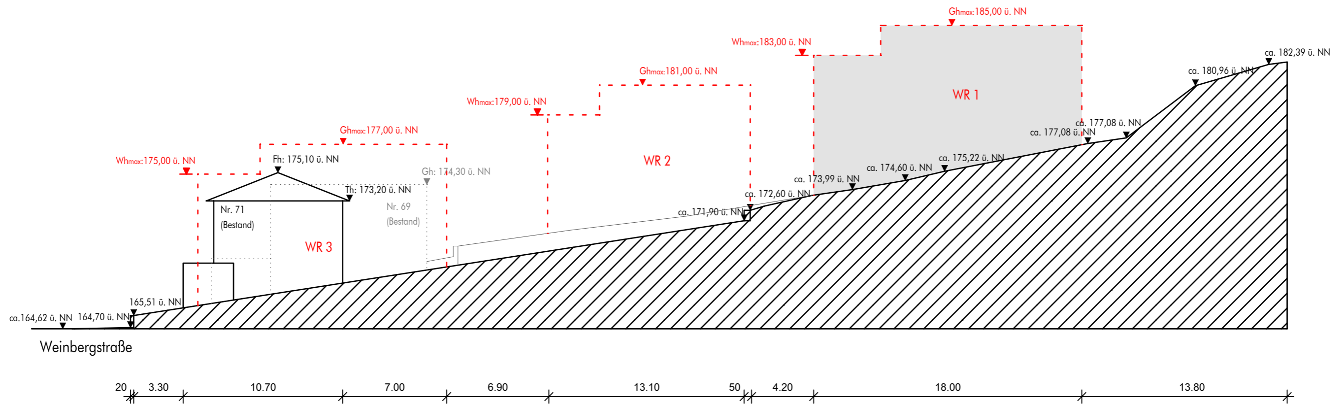
Schnitt B - B'
