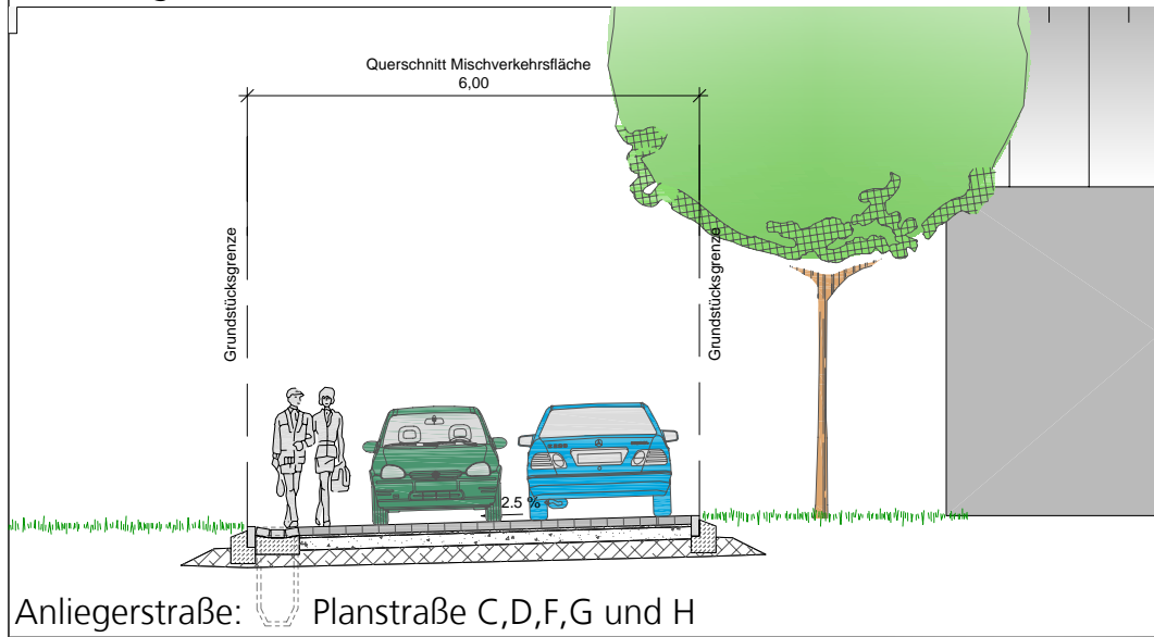
Anlage 2: Regelquerschnitte
