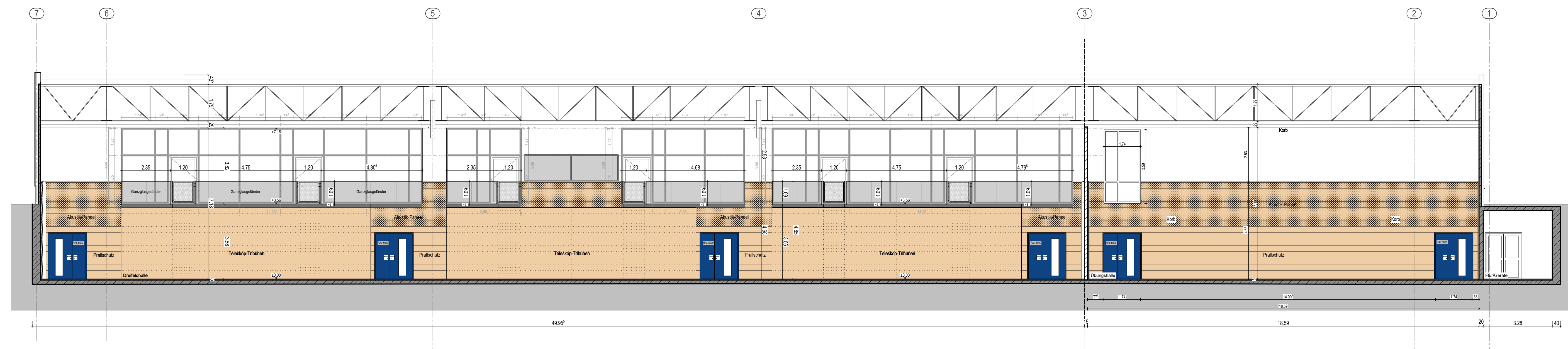
SCHNITT C-C - WANDABWICKLUNG OSTSEITE
