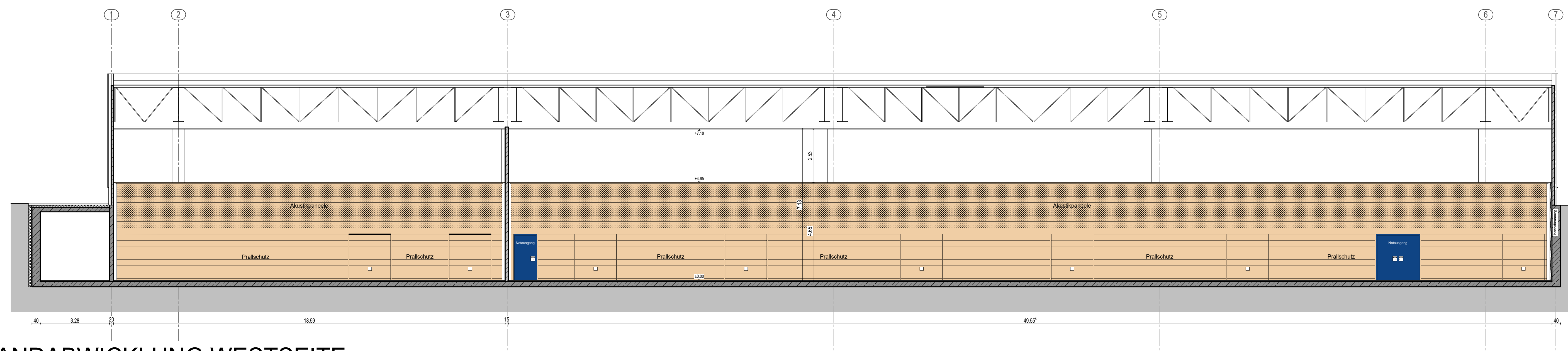
SCHNITT D-D - WANDABWICKLUNG WESTSEITE
